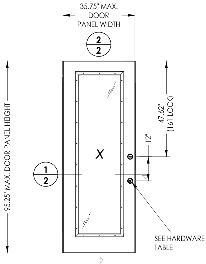
40 DOOR PANEL
